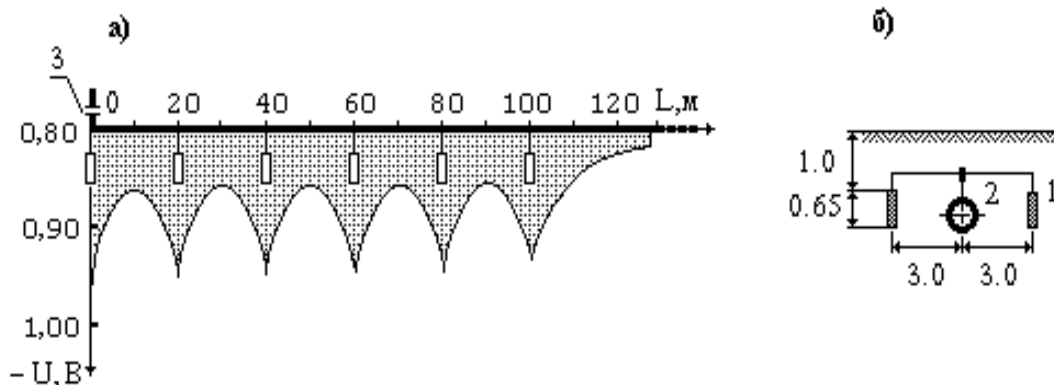
Рис.1. Графики разности потенциалов труба-земля (а) при протекторной защите трубопровода с установками по схеме (б): 1- протектор; 2 - трубопровод; 3 - изолирующее фланцевое соединение
