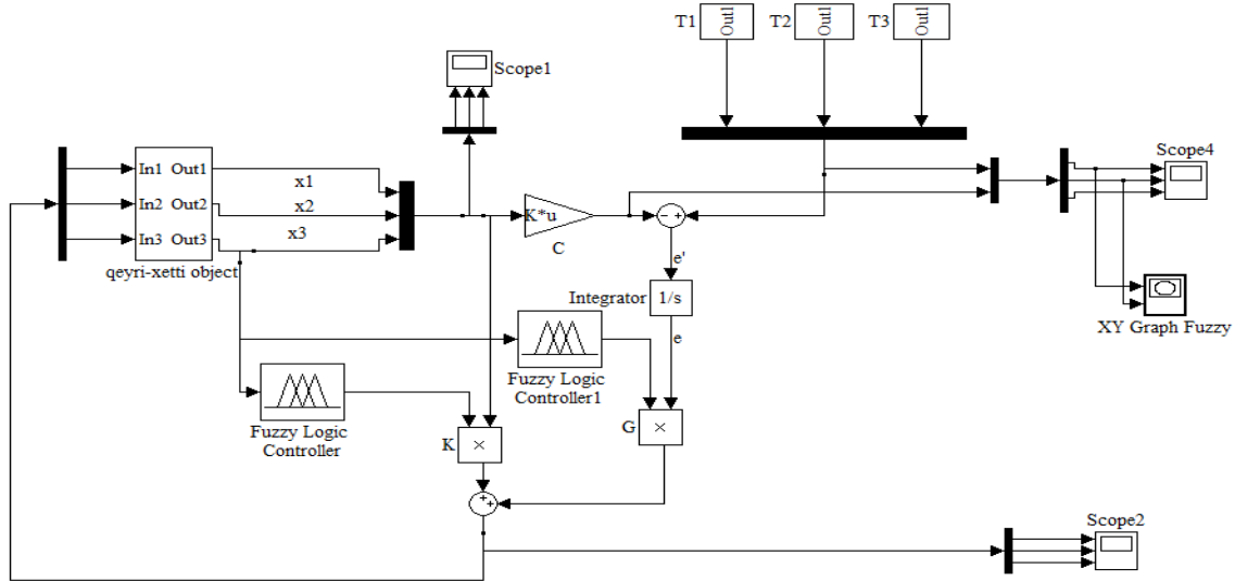
Şəkil 1. Mobil robotun robastlığı təmin edən idarəetmə sisteminin S- modeli
