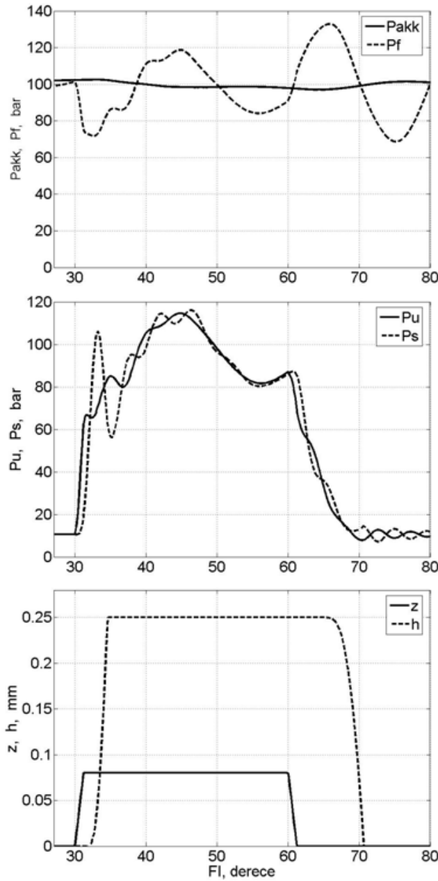
Şəkil 2. Təzyiq akkumulyatorundakı ( P_{akk} ), idarəedici klapanın həcmindəki ( P_f ), idarəetmə həcmindəki ( P_y ) və tozlandırıcının həcmindəki ( P_c ) yanacaq təzyiqinin və eləcə də pyezo-aktyuatorla idarəedici klapanın ( z ) və püskürdücü klapanın gedişinin ( h ) mühərrik valının dönmə bucağından ( F_i ) asılı olaraq dəyişmə əyriləri
