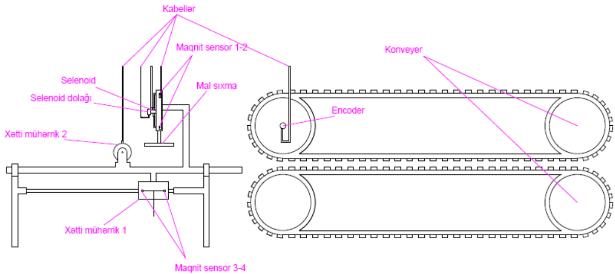
Şəkil 1. Kəsici qurğunun ümumi sxemi
