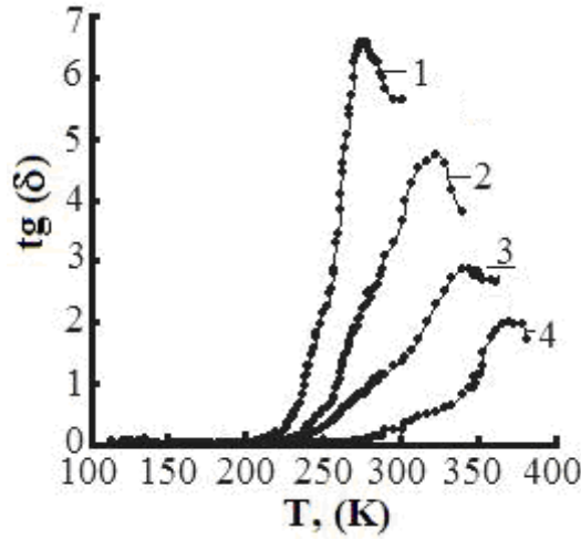
Şəkil 1. TlInTe 2 kristalı üçün dielektrik itgi bucağının tangensinin temperaturdan asılılığı. Ölçmələr aparılmış tezliklər: 1- 10; 2- 100; 3-500 və 1000 kHz
