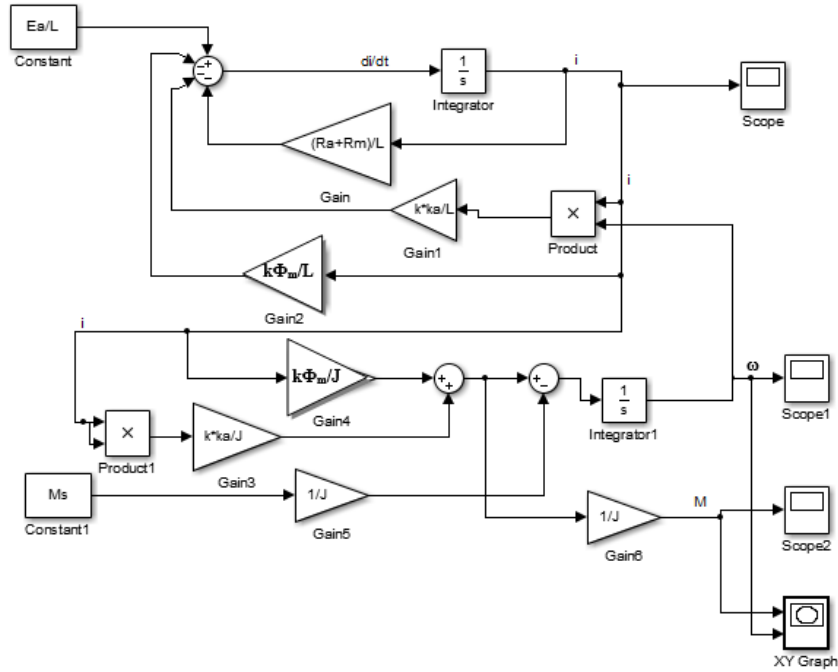
Şəkil 1. SCM-nin MATLAB/Simulinkdə tərtib edilmiş modeli
