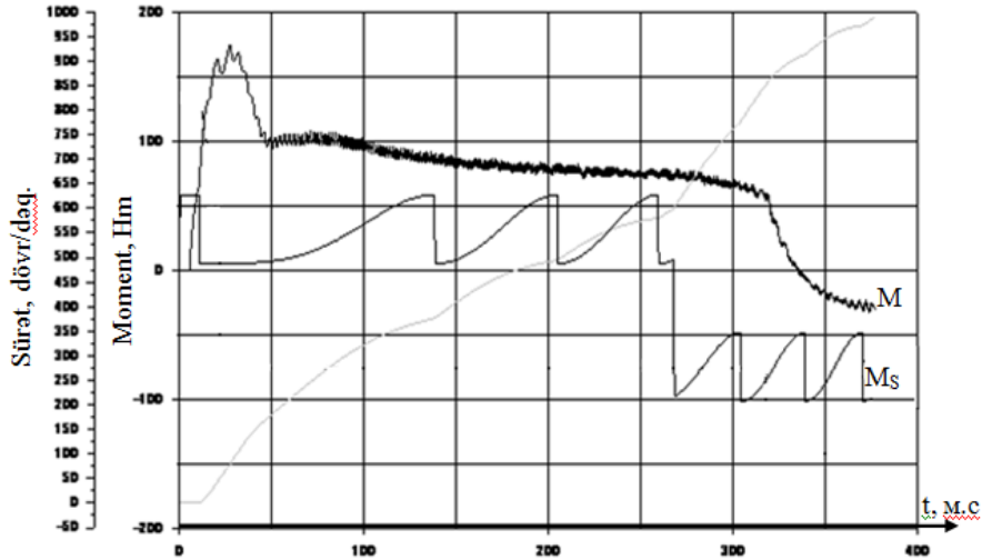
Şəkil 3. DYM-nin statik momentinin və sürətinin işəsalma prosesində qrafikləri
