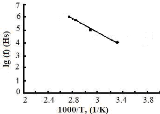
Şəkil 2. TlInTe 2 üçün dielektrik itgi bucağın tangensinin relaksasiya maksimumları tezliyinin temperaturun tərs qiymətindən asılılığı
