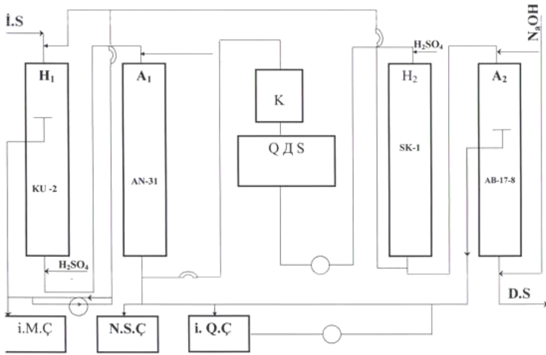
İlkin emalı zəruri olmayan (və ya koaqulyasiya edilmiş) təbii suların kimyəvi duzsuzlaşdırma sxemi.
