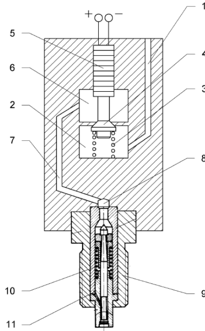
Şəkil 1. Elektron idarəetməli yeni konstruksiyalı forsunkanın prinsipial sxemi [1].
