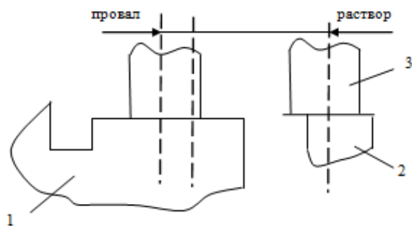
Рис. 2. Положение щеток в разных режимах 1 – коллектор; 2 – стойка; 3 – щетка.
