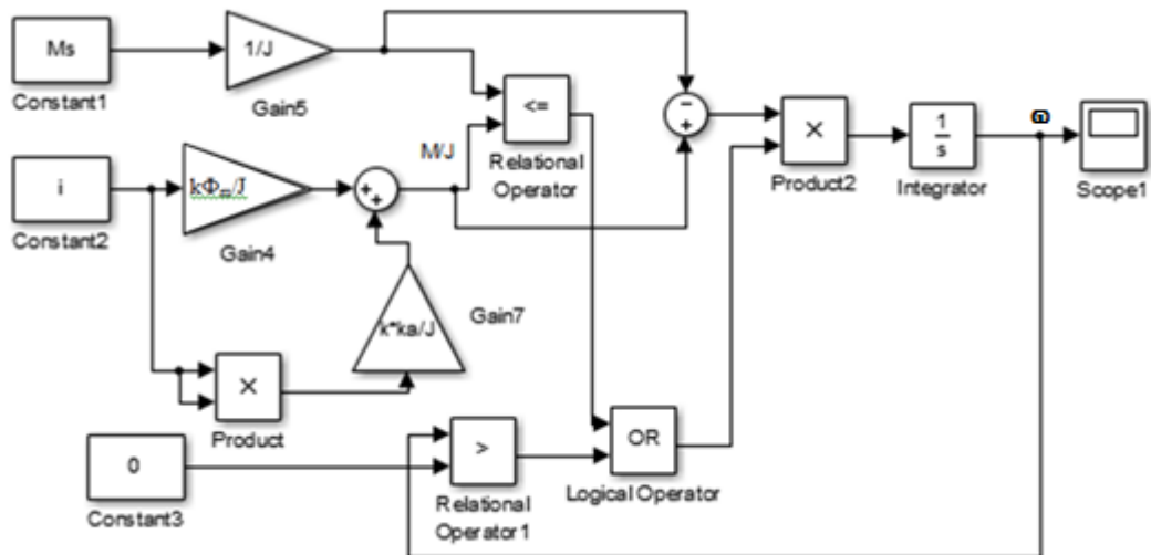
Şəkil 2. Reaktiv xarakterli statik momentin modeli
