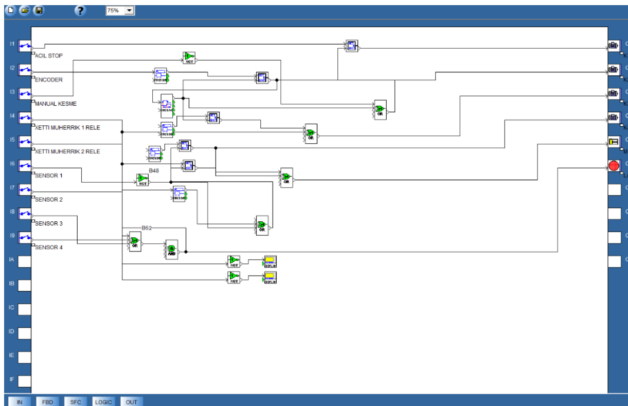
Şəkil 3. Kəsici qurğunun proqramı və işləmə prinsipi
