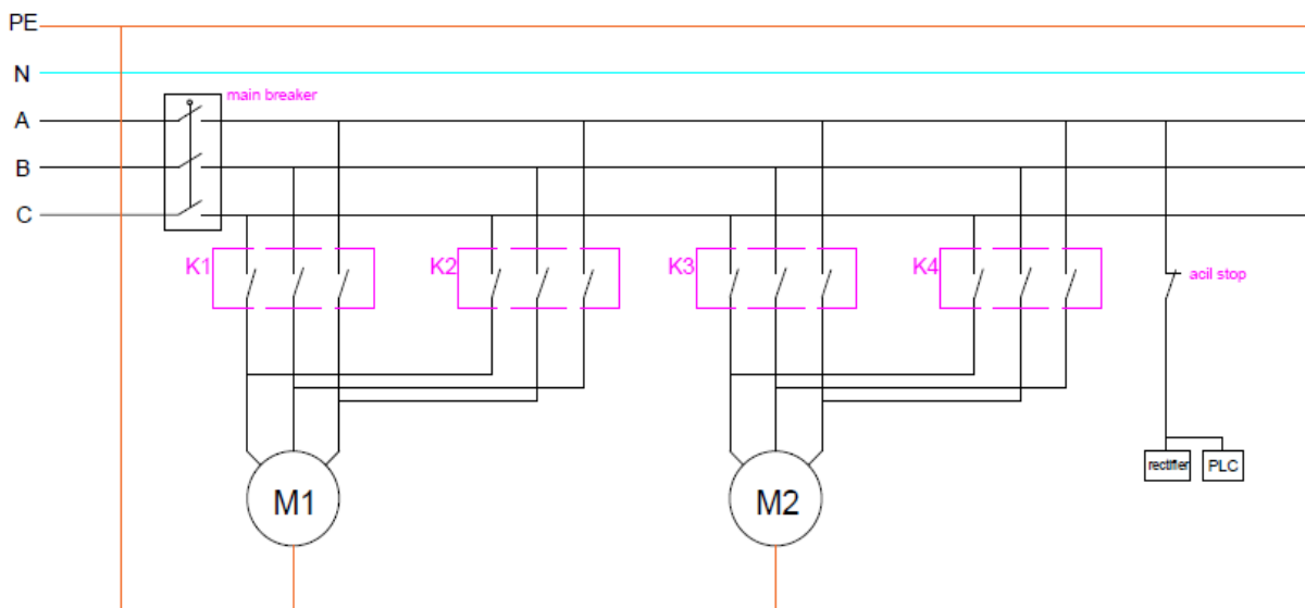
Şəkil 2. Kəsici qurğunun güc dövrəsi
