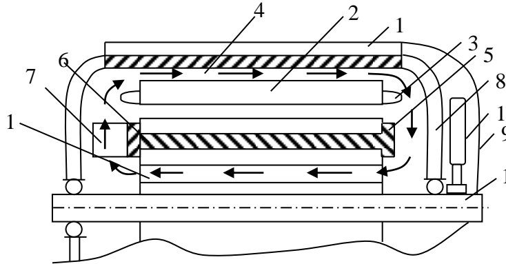
Şəkil 1. Mühərrikin konstruktiv ifası
