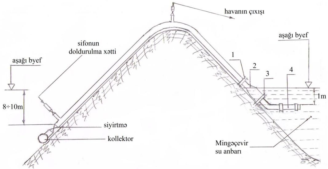
Şəkil 1. 1 - flyans birləşməsi, 2- yuxarı diametrə keçid, 3 - klapanı yerləşdirmək üçün xüsusi birləşmə, 4- suyu qəbul edən quruluş
