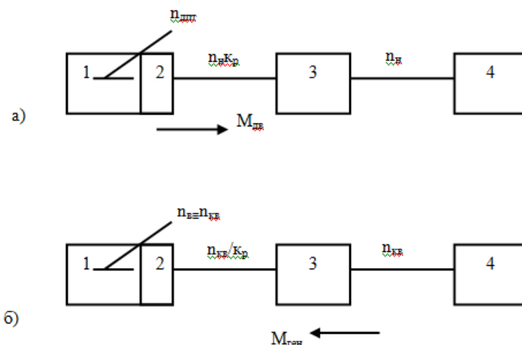
Рис. 1. Схема связи основных элементов стартер – генераторного комплекса
