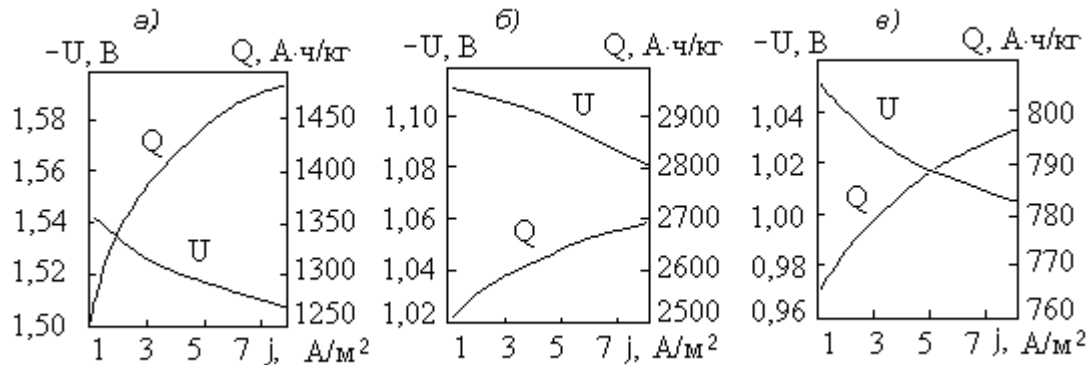
Рис.2. Изменение фактического потенциала ( U ) (по МЭС) и фактической токоотдачи ( Q ) сплавов МП1 (а), АП4 (б) и ЦП1,ЦП2,ЦП3 (в) с учетом плотности анодного тока
