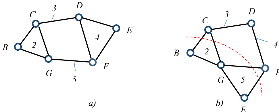
Şək. 3. a) Dördüncü sınıfa mənsub ikitərtibli Assur qrupu ( s=4, n=4, p=6, t=2, c=0 ); b) Sərbəstlik dərəcəsi sıfıra bərabər olan kinematik silsilə
