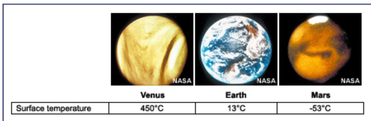
Şəkl.1. Bəzi planetlərin temperaturu: Venera, Yer, Mars
