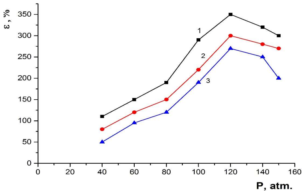
Şək. 2. Polietilen lövhələrinin deformasiya prosesi üzrə nəticələr
