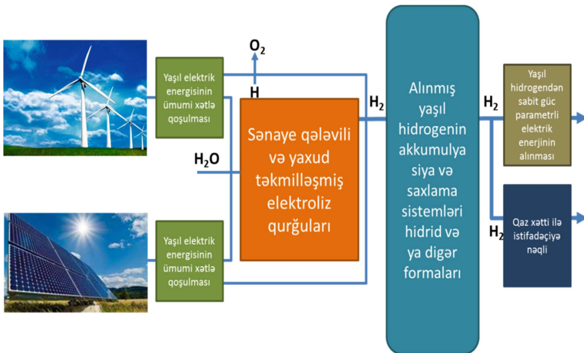
Şək. 2. Yaşıl Külək və Günəş enerjisinin dayanıqlı enerji mənbəyi kimi istifadəsi üçün kompleks texnologiyanın sxemi
