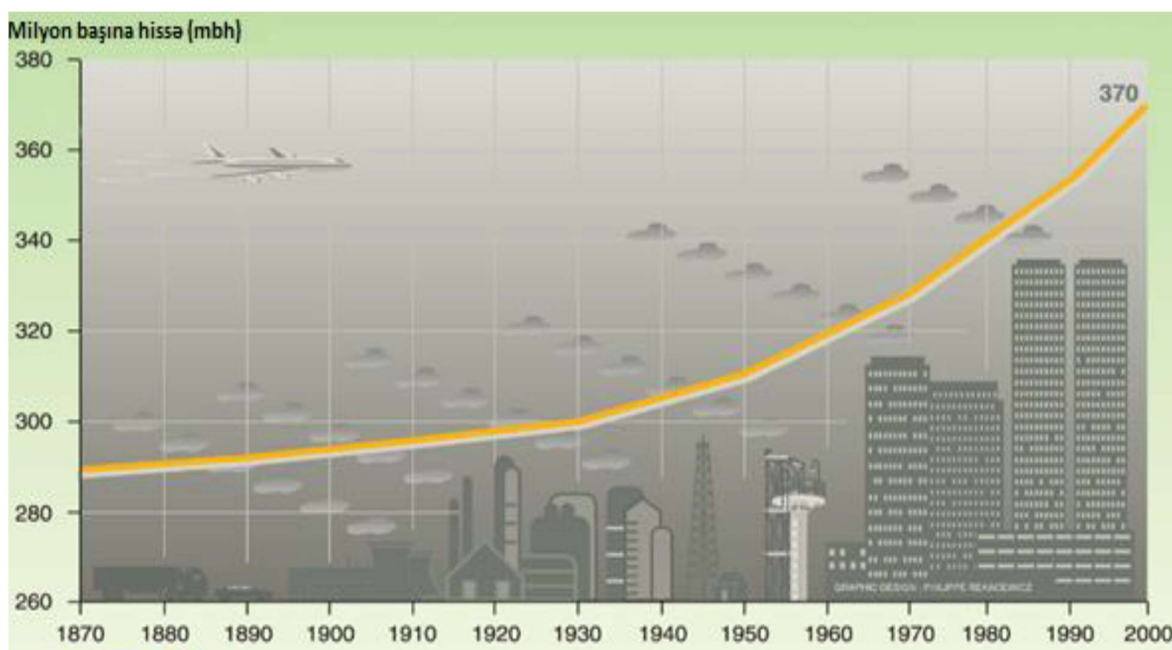
Şək. 1. Atmosferdə CO 2 –in qatılığının son 150 ildə dəyişmə kinetikasi
